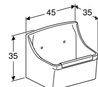
NORMA GOOTSTEEN
